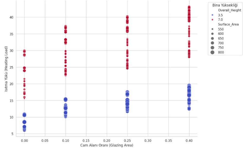
Mimari Parametrelerin Enerji Performansı Üzerindeki Etkisi
